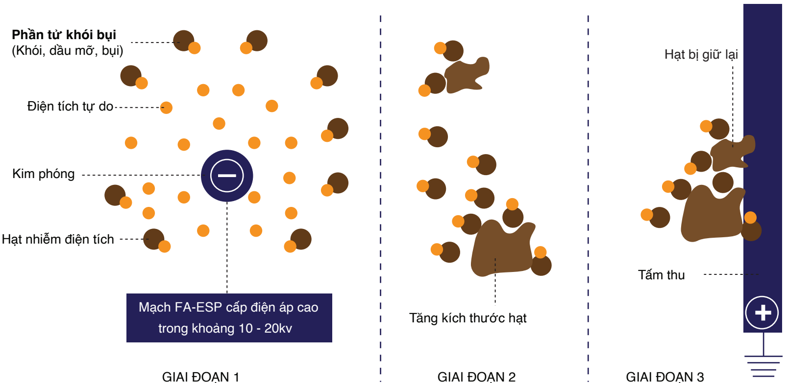
Mô phỏng giai đoạn xử lý khí thải bếp công nghiệp bằng FA-ESP
