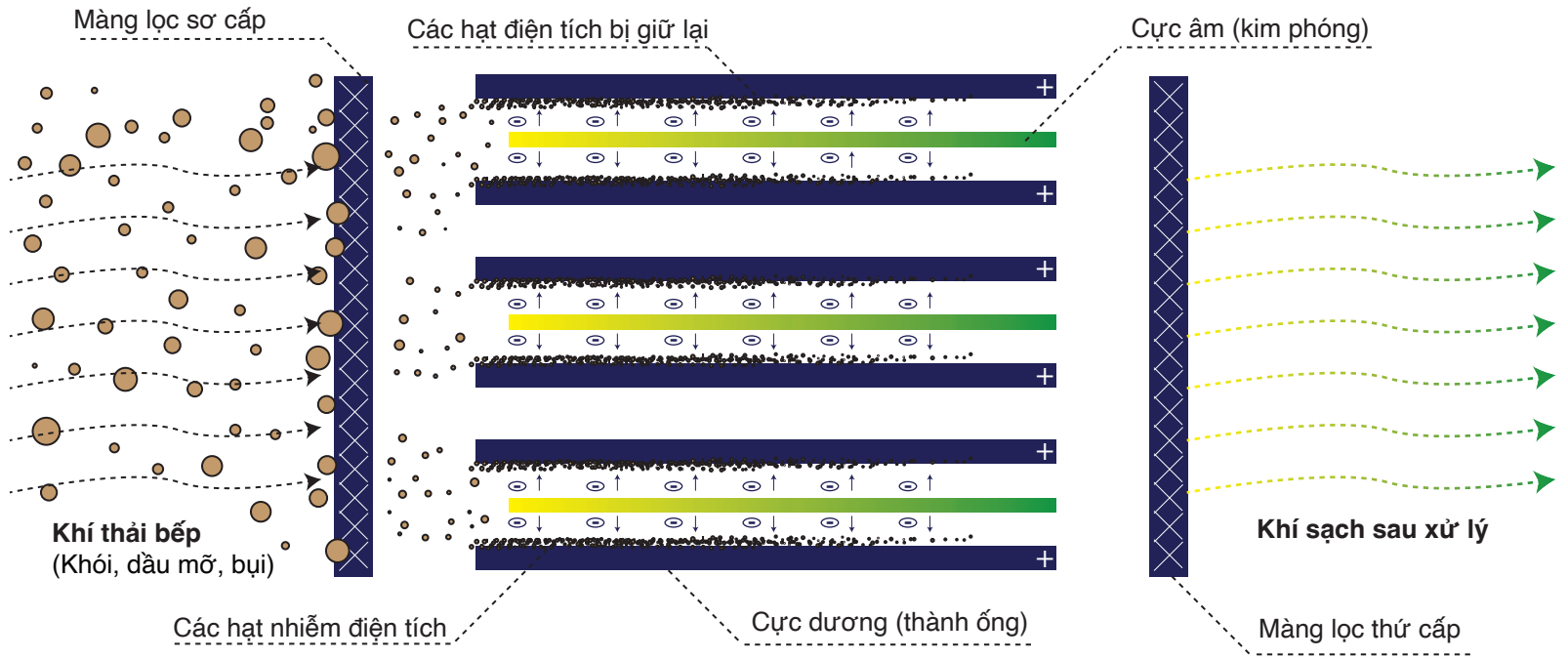
Mô phỏng quy trình xử lý máy lọc khói dầu tĩnh điện FA-ESP
