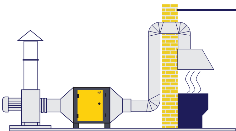
Lắp đặt hệ thống FA-ESP trên sàn
