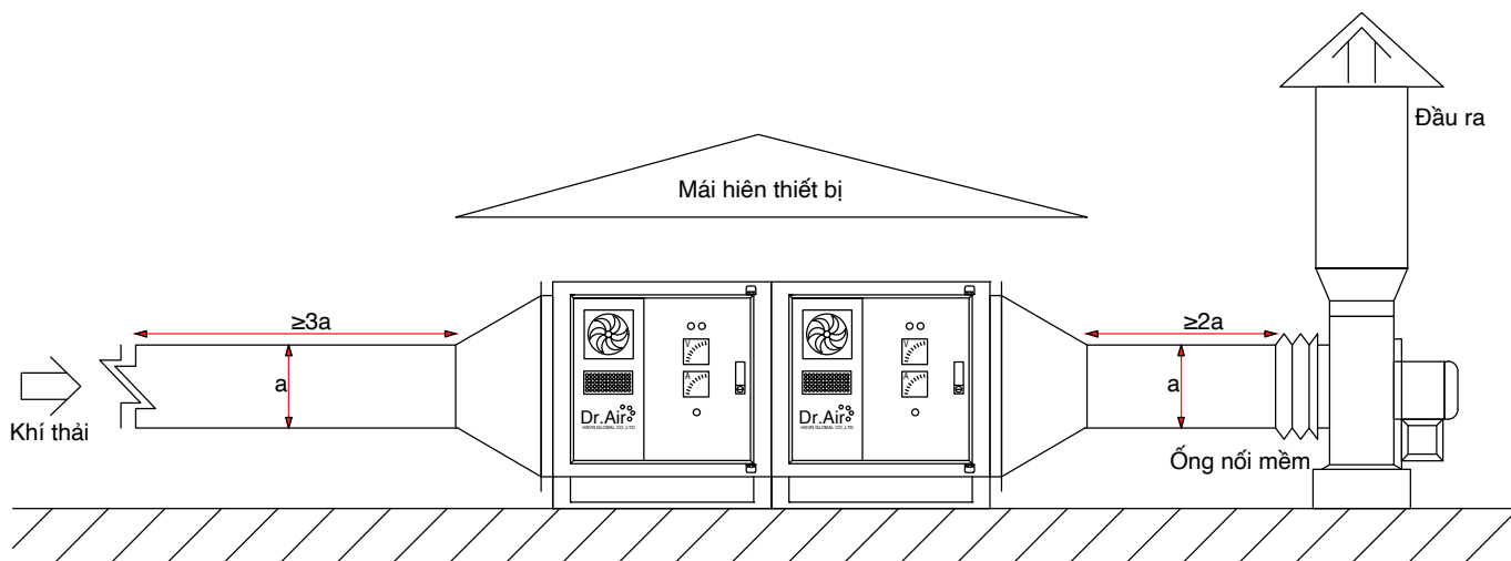
Mô hình lắp đặt máy lọc khói dầu tĩnh điện đúng cách
