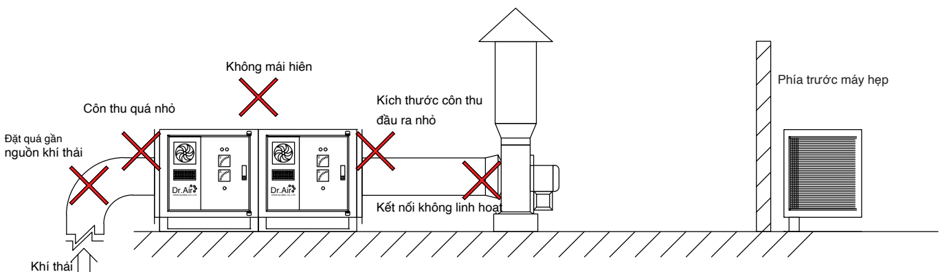
Những lỗi thường gặp & nên tránh khi lắp đặt máy lọc khói dầu tĩnh điện
