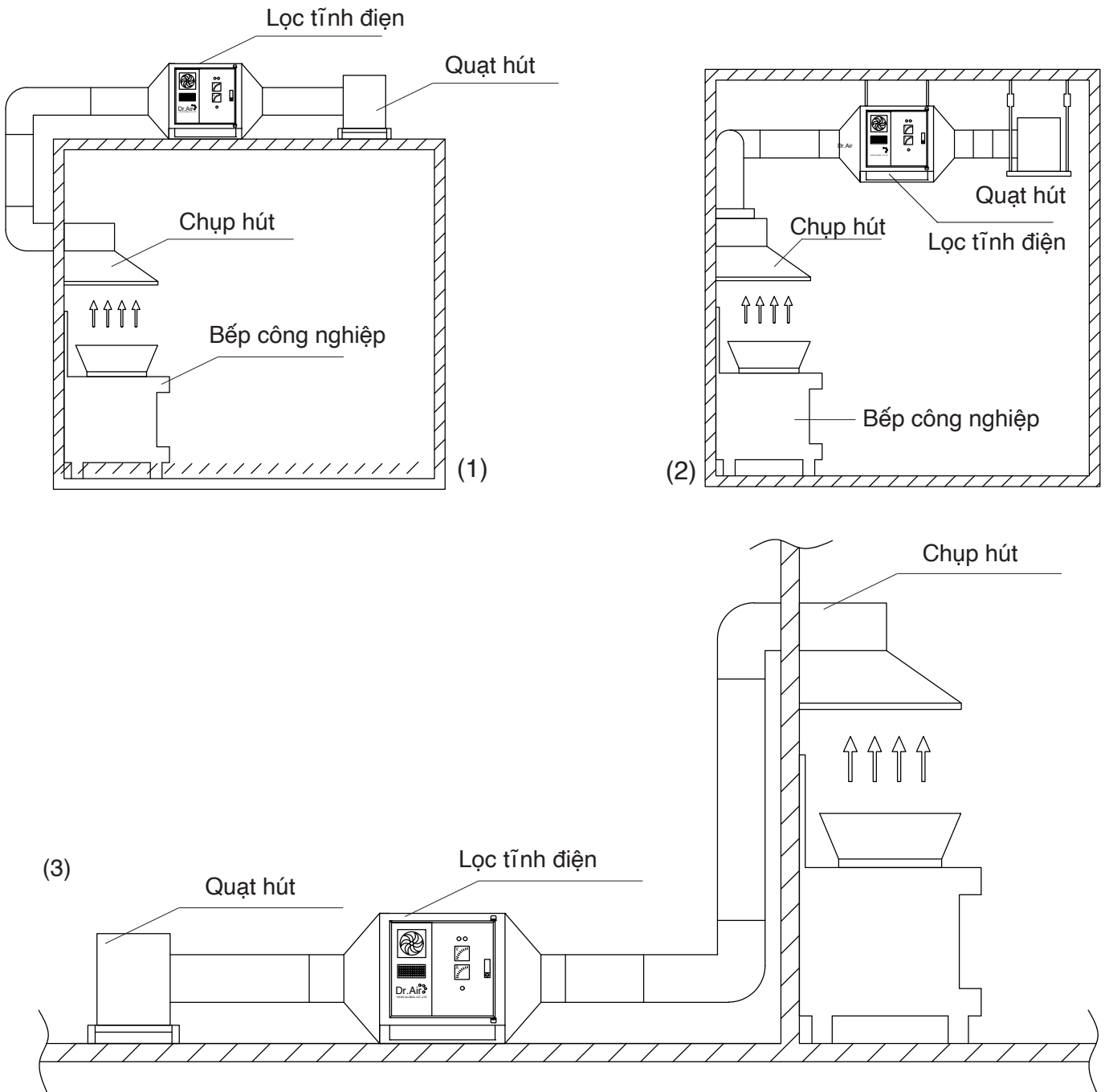
Mô hình lắp đặt máy lọc khói dầu tĩnh điện Dr.Air KT
